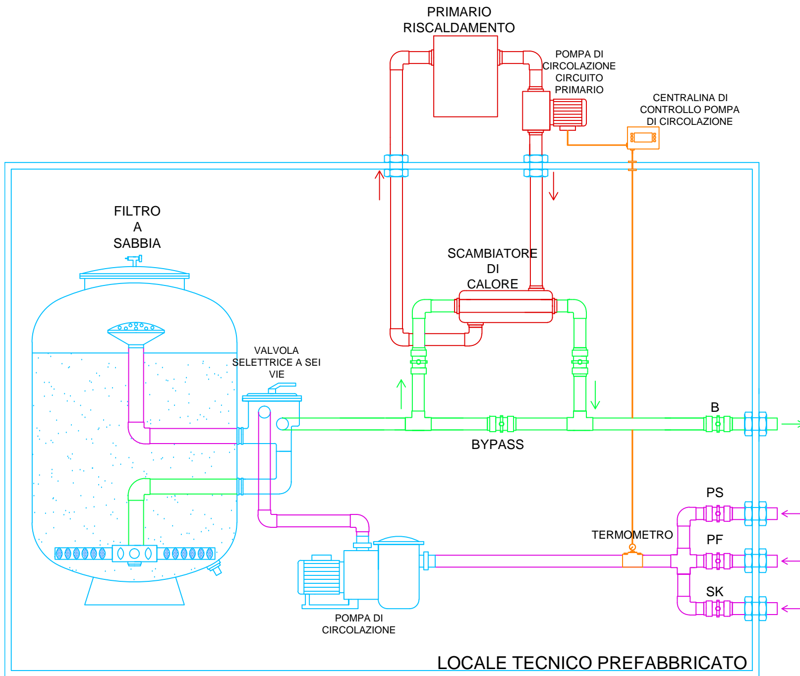
ACQUA SPA SCHEMA INSERIMENTO RISCALDAMENTO CON SCAMBIATORE DI CALORE
