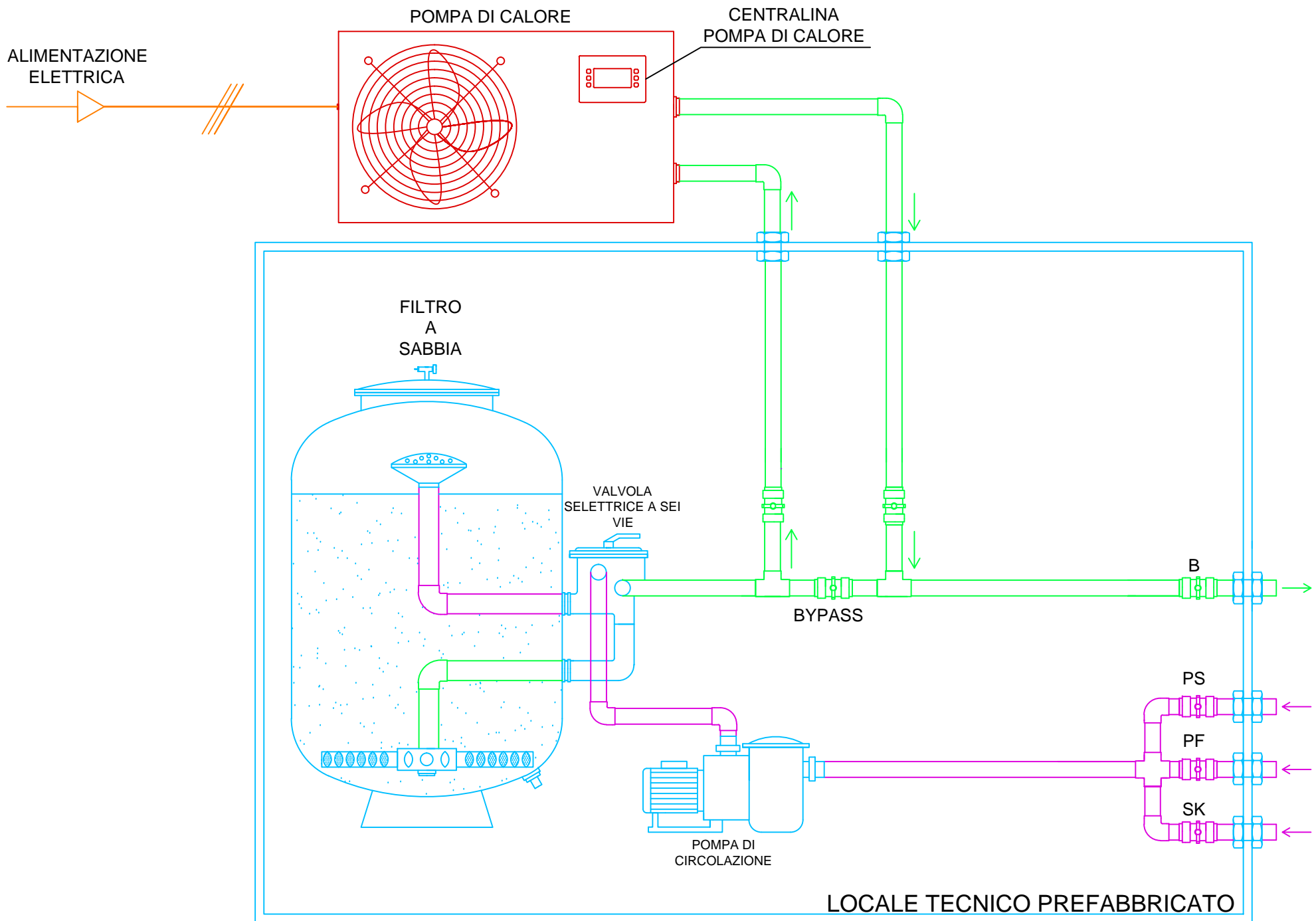
ACQUA SPA SCHEMA INSERIMENTO RISCALDAMENTO CON POMPA DI CALORE
