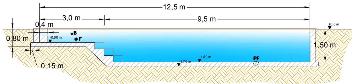
SEZIONE A-A'
