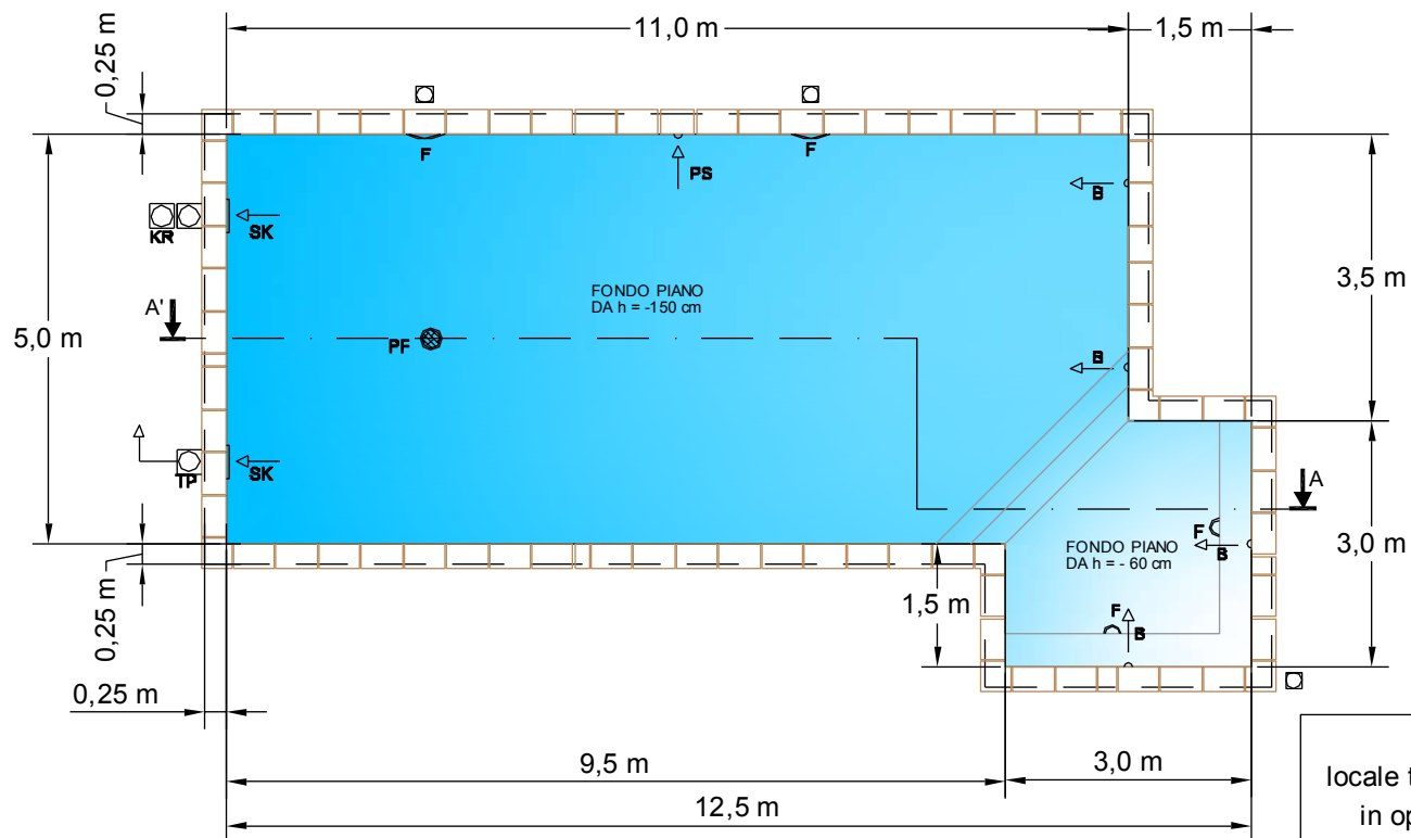
PIANTA
