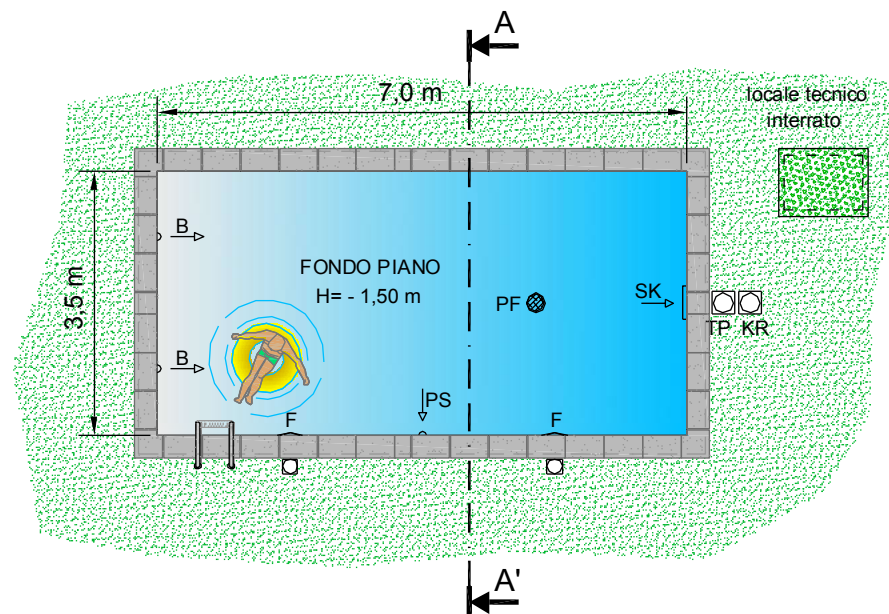
PIANTA
