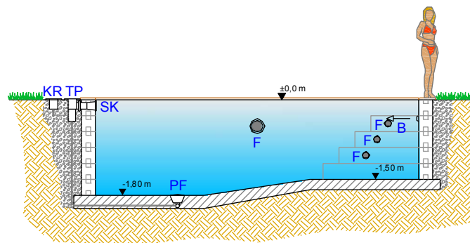
SEZIONE A-A'
