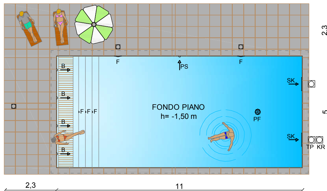
PIANTA
