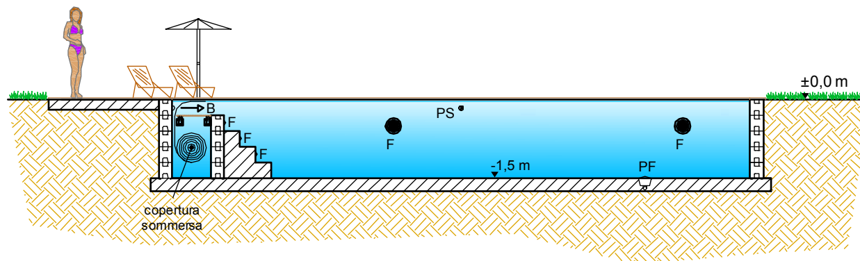
SEZIONE
