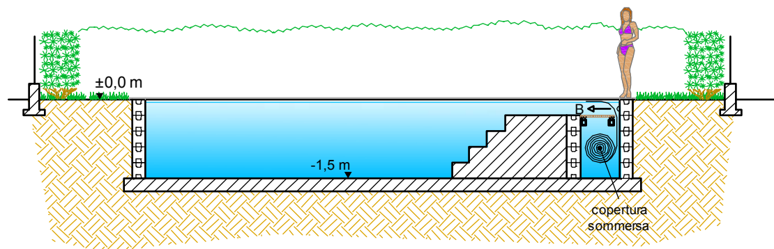
SEZIONE
